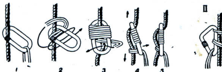
Рис. 19. Два варианта схватывающего узла на карабине
